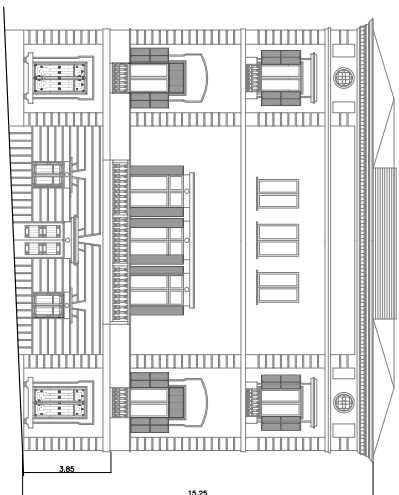
FAÇANA POSTERIOR PL. DE L'AJUNTAMENT
