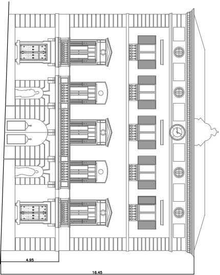
FAÇANA PRINCIPAL LA RIERA
