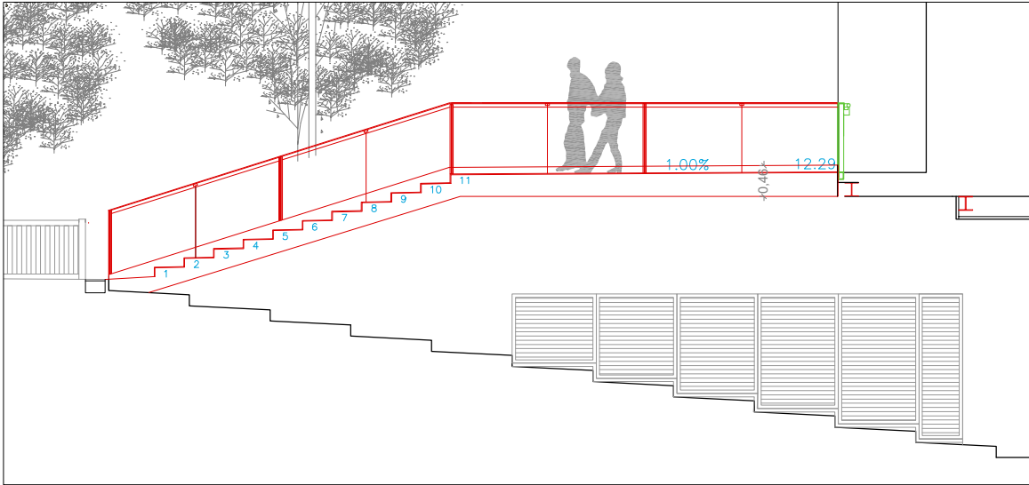
SECCIÓ A-A' ESTAT PROJECTAT
