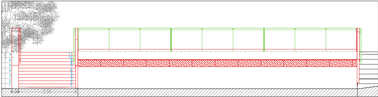
SECCIÓ B-B' ESTAT PROJECTAT
