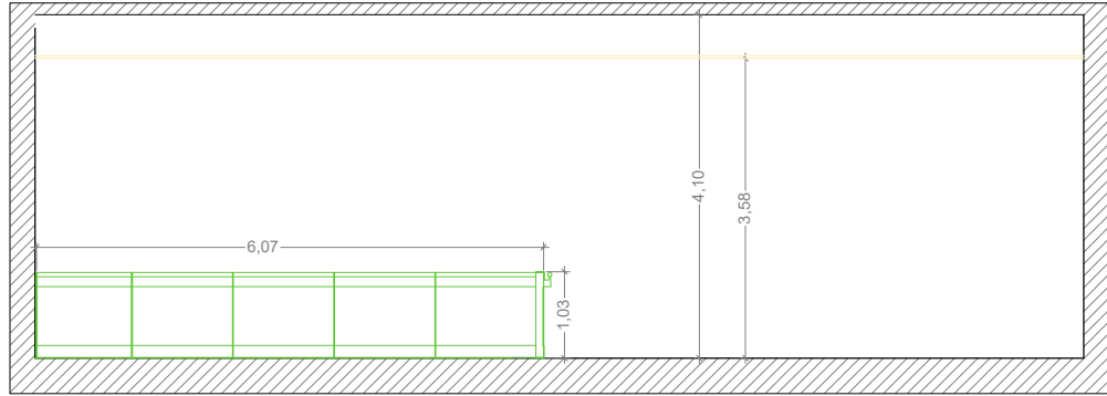
SECCIÓ G-G' ACTUAL
